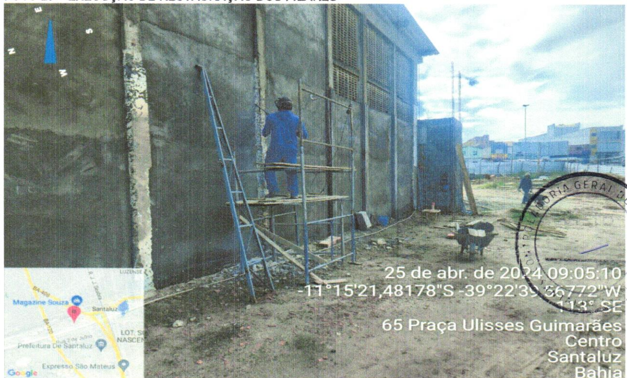
FOTO 28 – EXECUÇÃO DE RESTAURAÇÃO DOS PILARES
