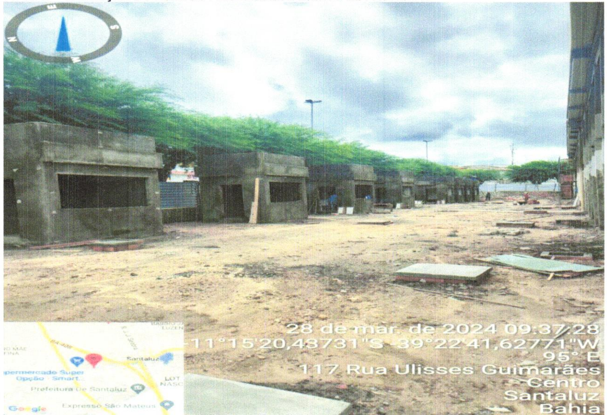
FOTO 18 - CAIXA DE DRENAGEM TIPO I - DIMENSÕES 0,80X0,80X1,00M
