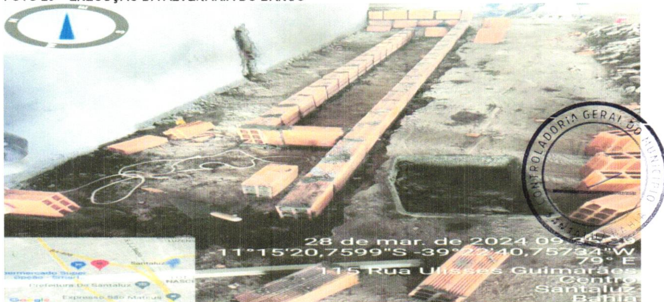
FOTO 20 - EXECUÇÃO DA ALVENARIA DO BANCO
